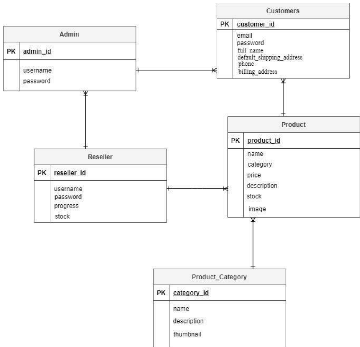
Figure 46: ER Diagram
